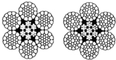
G IWRC 6xWS(31) G IWRC 6xWS(36)
